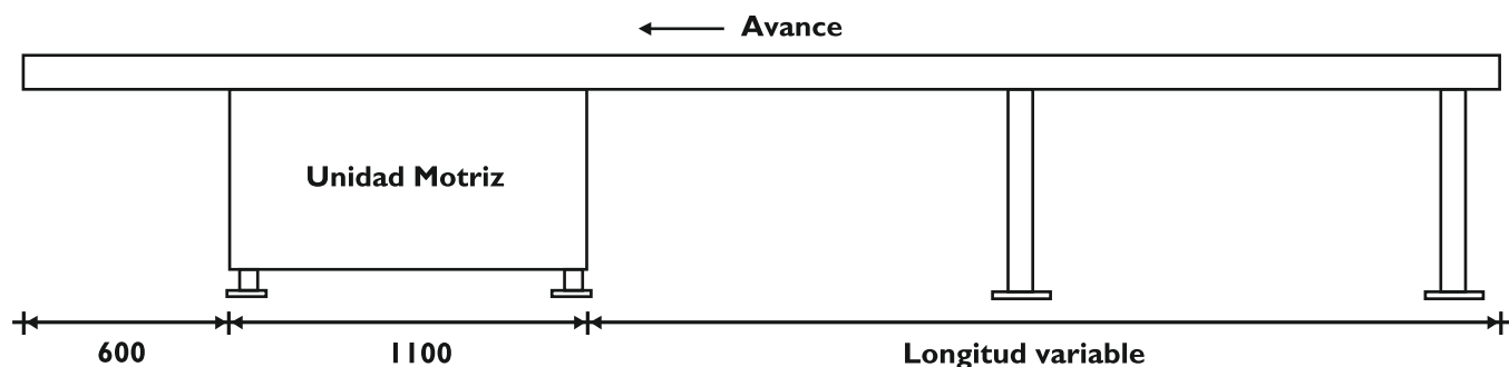
Modelo TRF Un Transportador para Charolas diseñado especialmente para usted.
